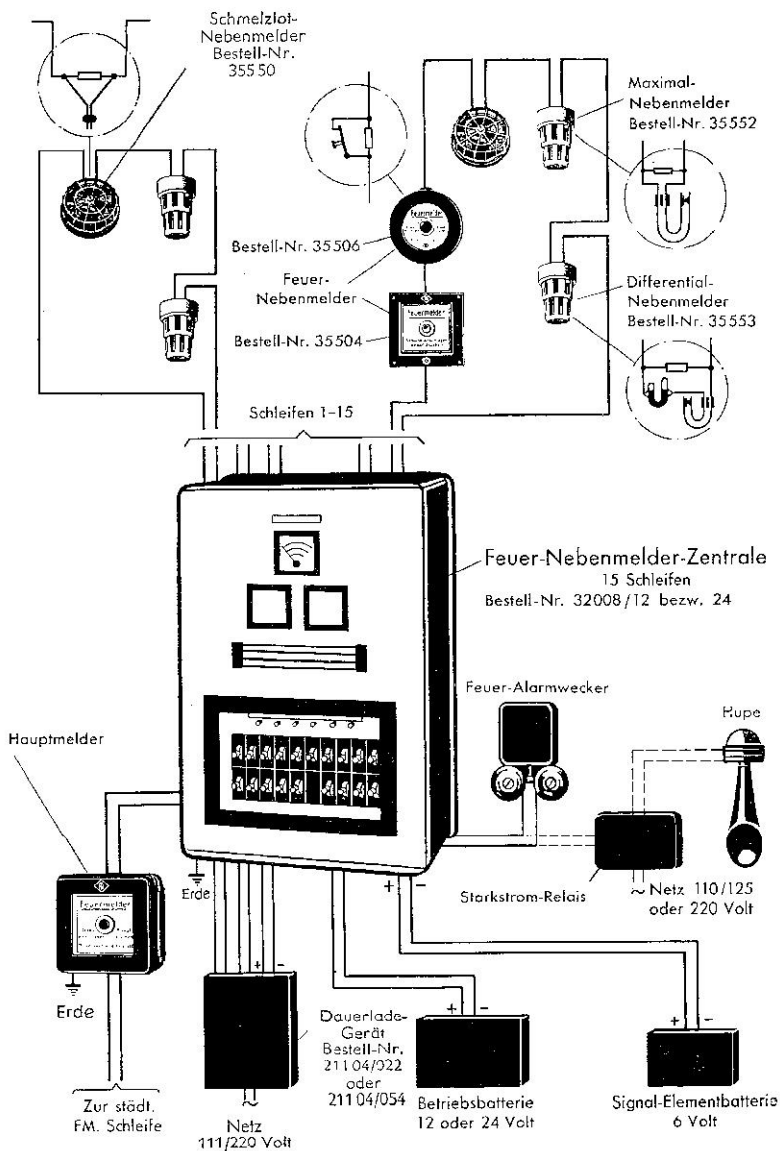
Prinzipdarstellung einer Feuer-Nebenmelder-Anlage nach dem Stromschwächungsprinzip 12 oder 24 Volt Betriebsspannung
